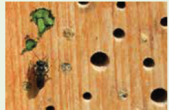
Bild 3: verschlossene Nisthöhlen
